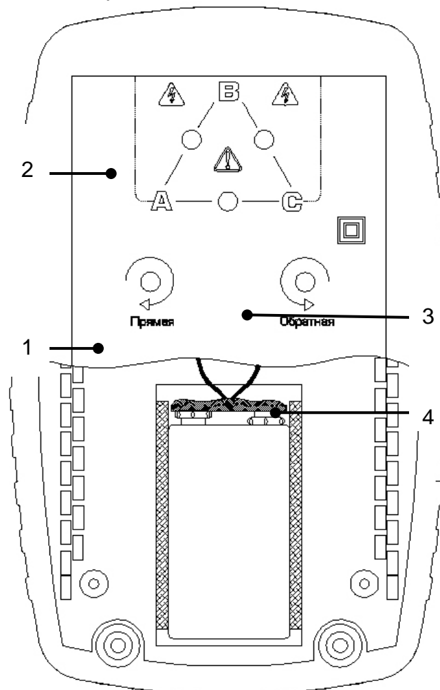
Рисунок 4.2 – Расположение батареи в указателе
