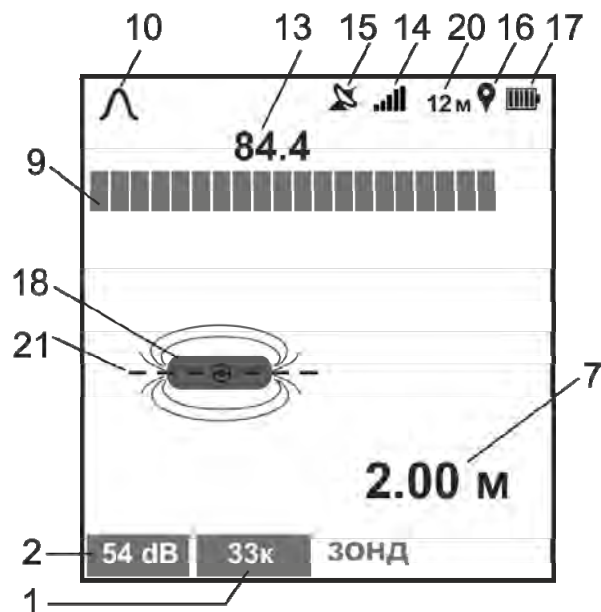
Рисунок 3.4 – Индикация приемника в режиме «ЗОНД»
