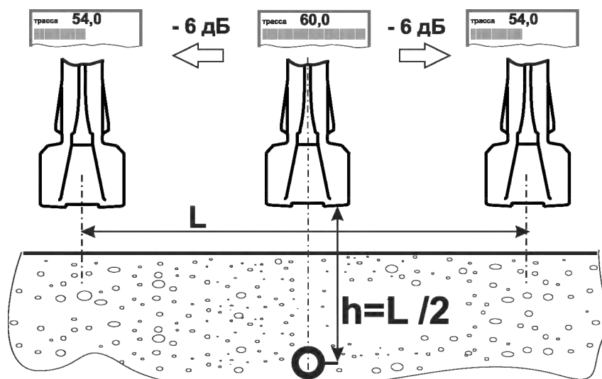
Рисунок 4.3.1 – Определение глубины залегания методом «-6дБ»
