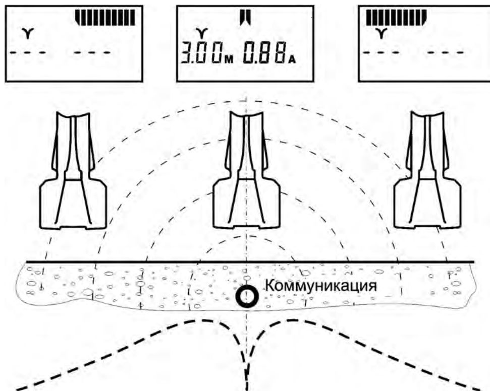
Рисунок 3.2.2 – Изменение уровней сигналов при смещении приёмника относительно оси коммуникации
