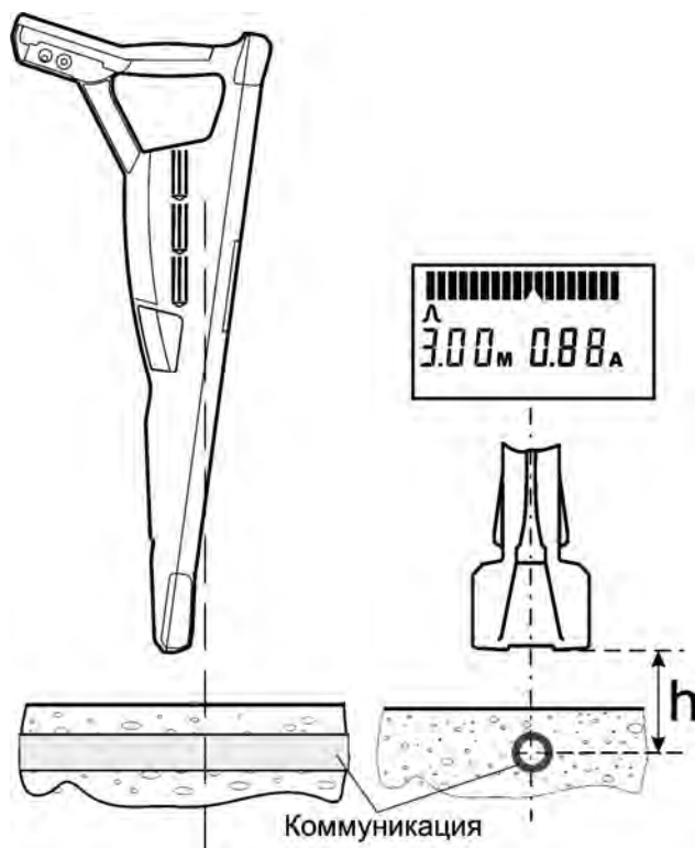
Рисунок 3.3.1 – Прямое определение глубины залегания
