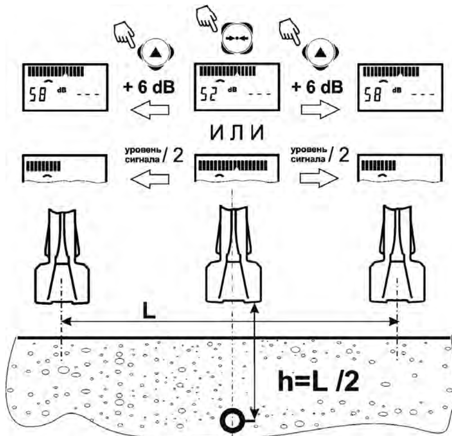
Рисунок 3.3.2 – Определение глубины залегания косвенным методом
