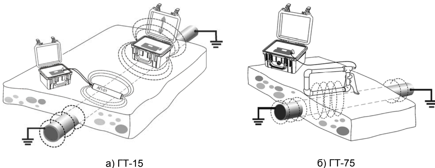
Рисунок 2.3.2 – Способы бесконтактного задания тока в коммуникации
