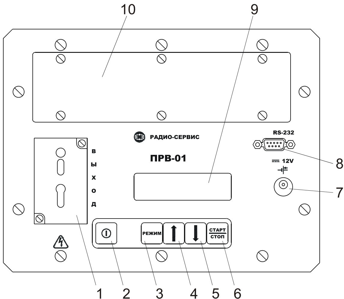
Рисунок 1 – Лицевая панель прибора
